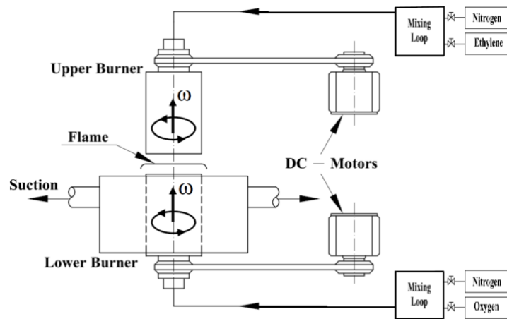
圖 1. 旋轉對沖流擴散火焰燃燒器。
